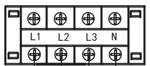
Клеммная колодка наружного блока
