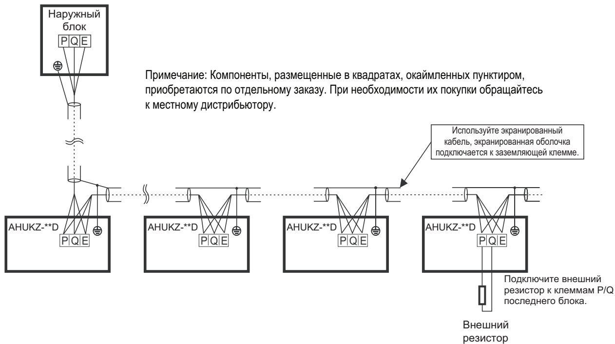
Организация схемы управления
