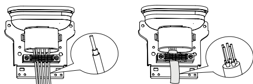
Метод закрепления 1: зажим для проводов на силовом кабеле
