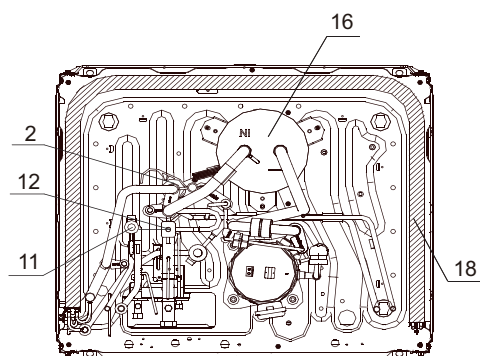
Условные обозначения № Наименование детали 1 Компрессор 2 Сепаратор масла 3 Реле высокого давления 4 Обратный клапан 5 Датчик высокого давления 6 Вентилятор 7 Микроканальный теплообменник 14 Запорный вентиль (труба газовой линии) 9 Электронный расширительный вентиль (EEVA) 8 Запорный вентиль (жидкостная труба) 11 Электронный расширительный вентиль (EEVC) 10 Порт для заправки 13 Электронный расширительный вентиль (ЭРВ по заказу) 15 Датчик низкого давления 16 Газожидкостный сепаратор 17 Глушитель 18 Теплообменник
