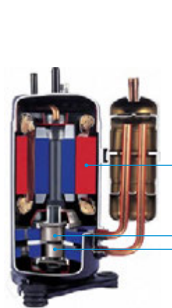
Конструкция двухроторного компрессора производства Mitsubishi Electric
