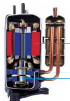
Компрессор (двухроторный)
